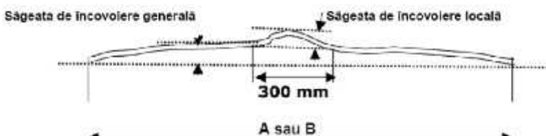
Figura 2 – săgeata de încovoiere generală și săgeata de încovoiere locală
